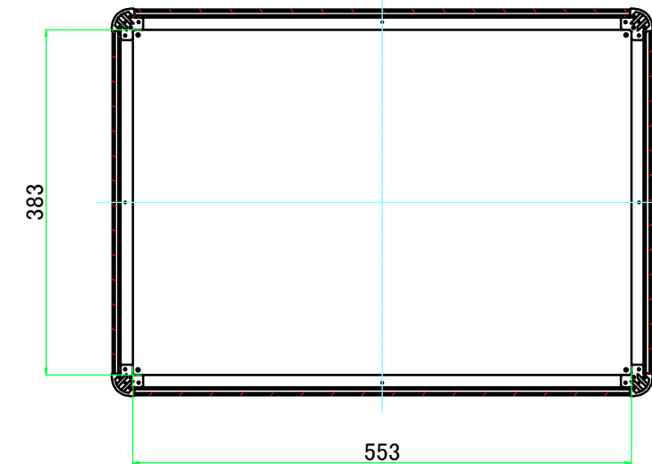
C-C ( 1 : 7.5 )
