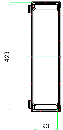
B-B ( 1 : 7.5 )
