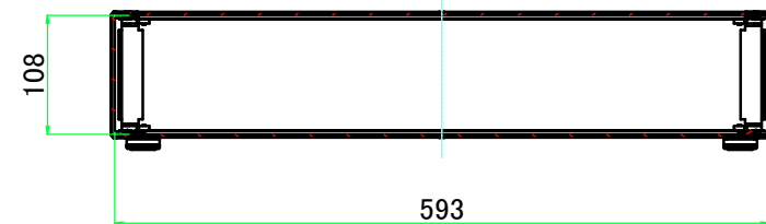
A-A ( 1 : 7.5 )
